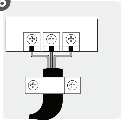
Sluit de bedrading aan. (Niet van toepassing op sommige locaties in Noord-Amerika.)
