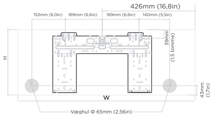
Indendørs enhedens dimensioner (BxH): 812mm(40,0in)x299mm(11,8in)
