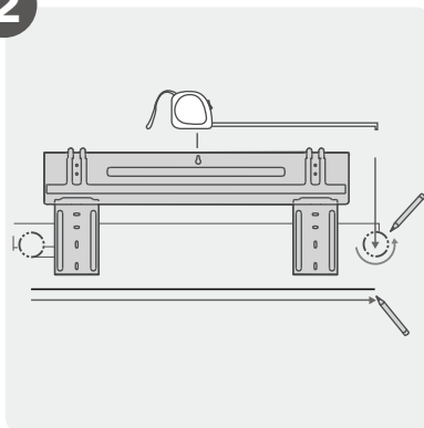
Fixer la plaque de montage
