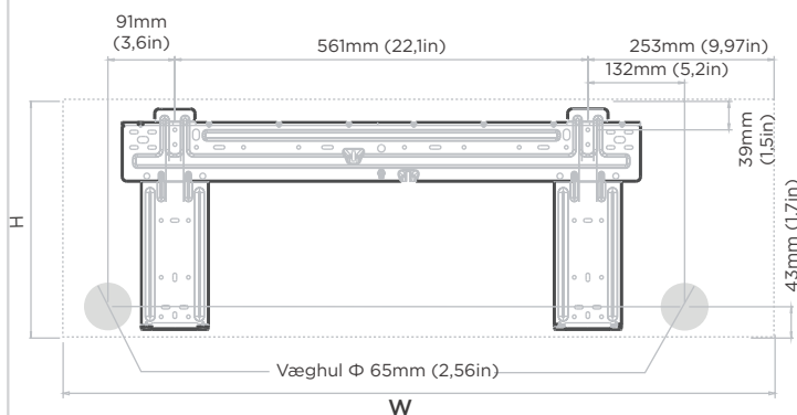
Indendørs enhedens dimensioner (BxH): 968mm(38,1in)x322mm(12,7in)
