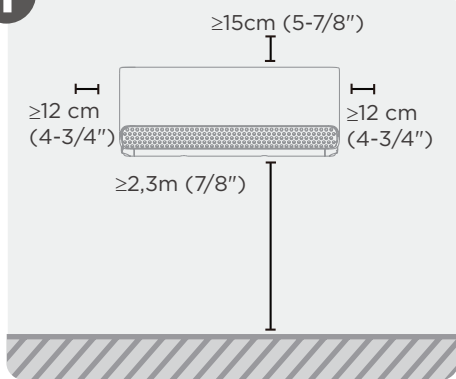
Vælg installationsplacering
