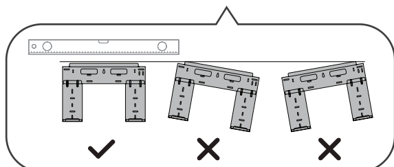
Corretto orientamento della piastra di montaggio
