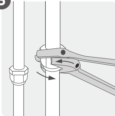
Tilslut rørledning
